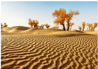
土地荒漠化
