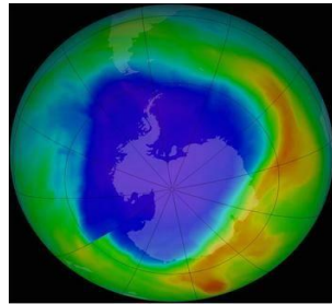
臭氧层破坏
